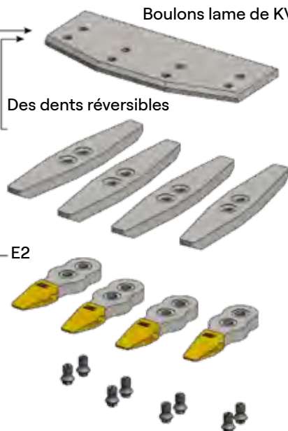
Boulons lame de KVVX
